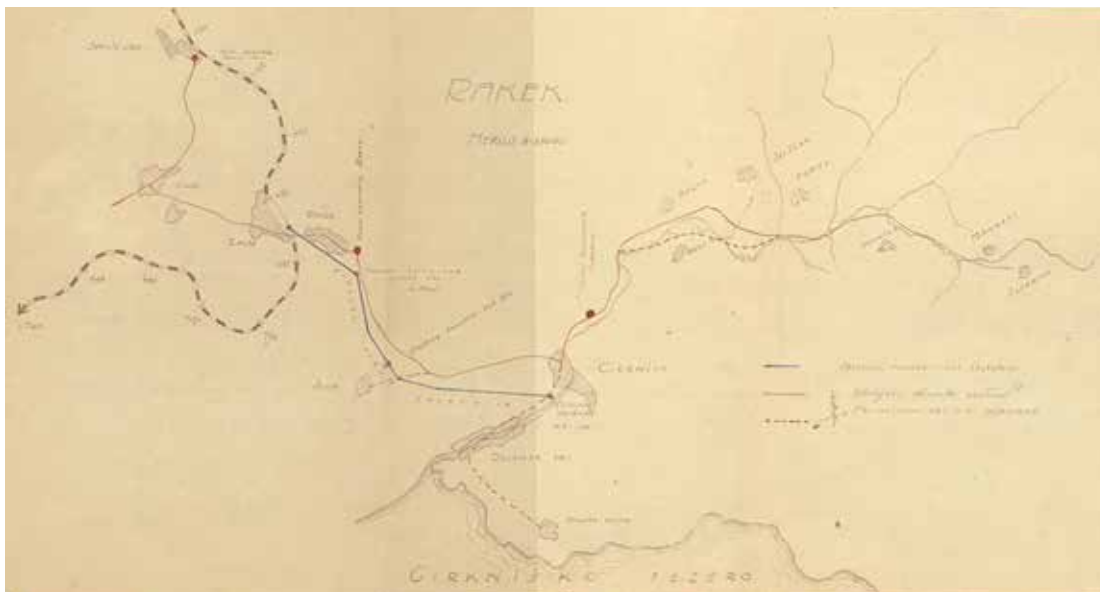
Na malo slabše vidnem zemljevidu je narisana potek vodovoda od zajetja vodovoda do postaje na Rakeku. Nad cesto Cerknica–Begunje nad Krajcevo žago je narisana vodni rezervoar. Avtor: neznan Zbirka: Karel Rustja
